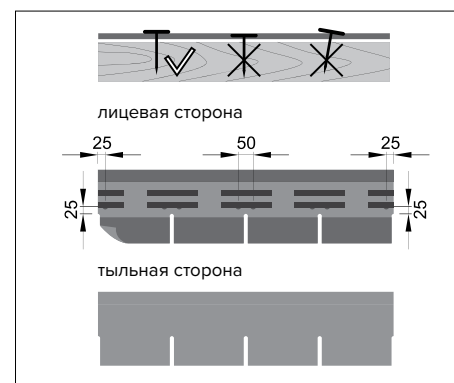
Рис. 1.1. Схема крепления фасадной плитки
