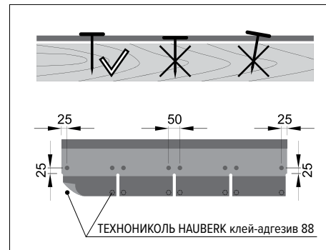
Рис. 1.1. Схема крепления фасадной плитки
